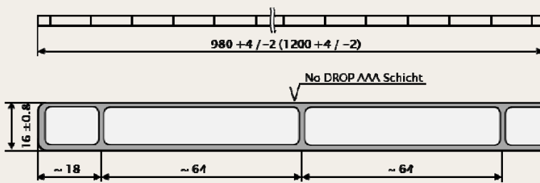
Querschnitt der PLEXIGLAS® Resist AAA SDP 16-64 (Maße in mm)
